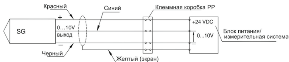
Рисунок 3 – Схема электрических подключений преобразователей модификаций PC-SG-25, PC-SG-25S с выходным сигналом от 0 до 10 В
