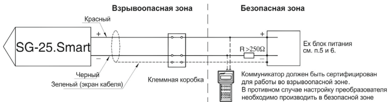
Рисунок 2 – Схема электрических подключений преобразователей модификаций PC-SG-25.Smart, PC-SG-25S.Smart в Ex исполнении
