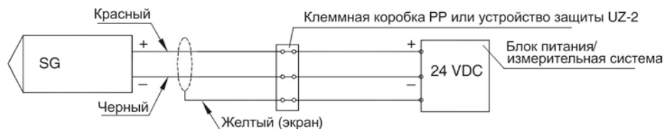
Рисунок 4 – Схема электрических подключений преобразователей модификаций PC-SG-25, PC-SG-25S с выходным сигналом от 4 до 20 мА, от 0 до 5 мА
